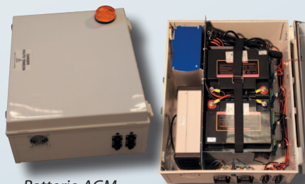
Batterie AGM
